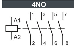
Bağlantı Şeması:
